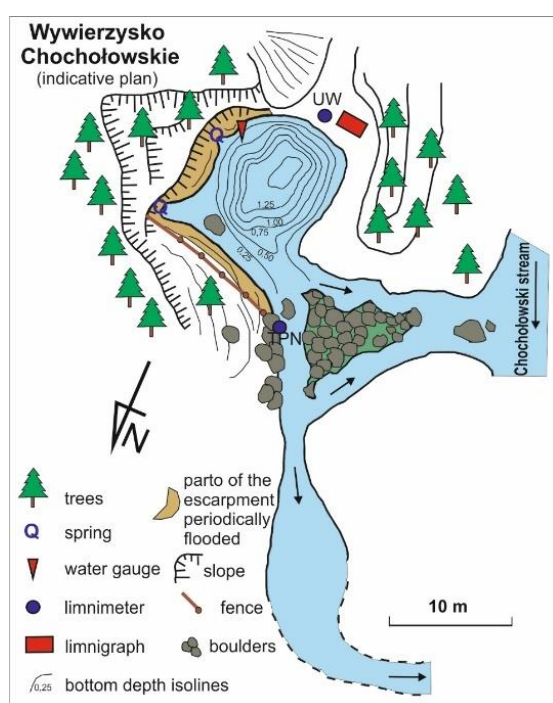
Plan of the Wywierzysko Chocholowskie (after Barczyk 2008)
