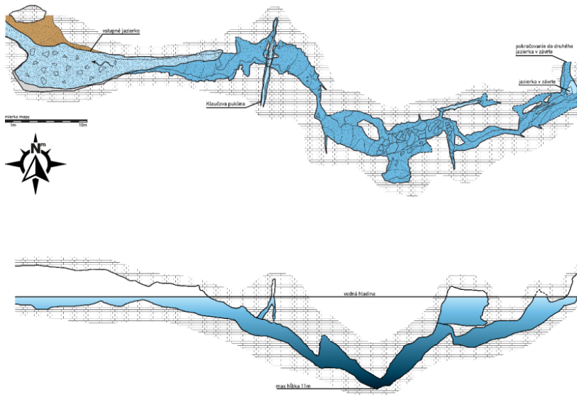
Cave map of the Brestovská vyvieračka spring.
